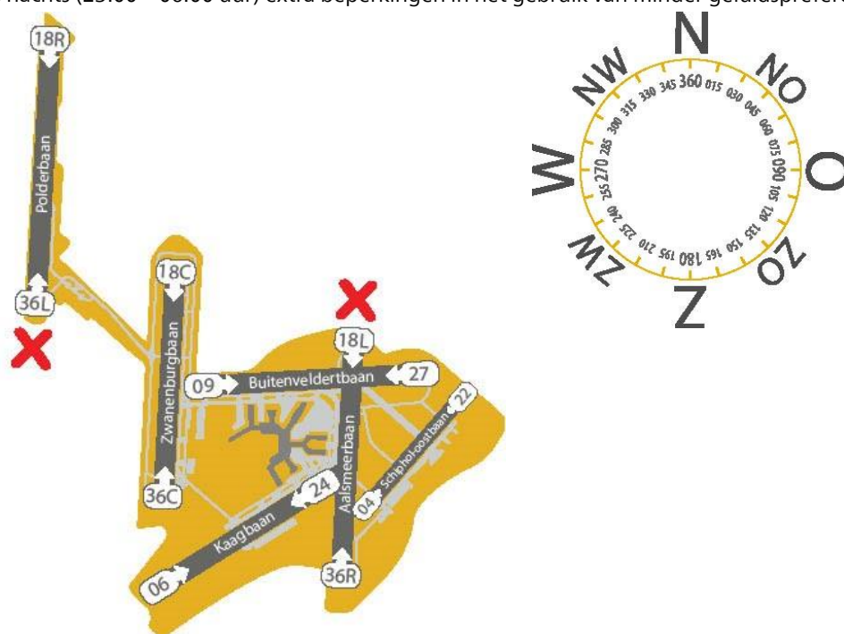
Figuur 4.1: Banenstelsel Schiphol.
